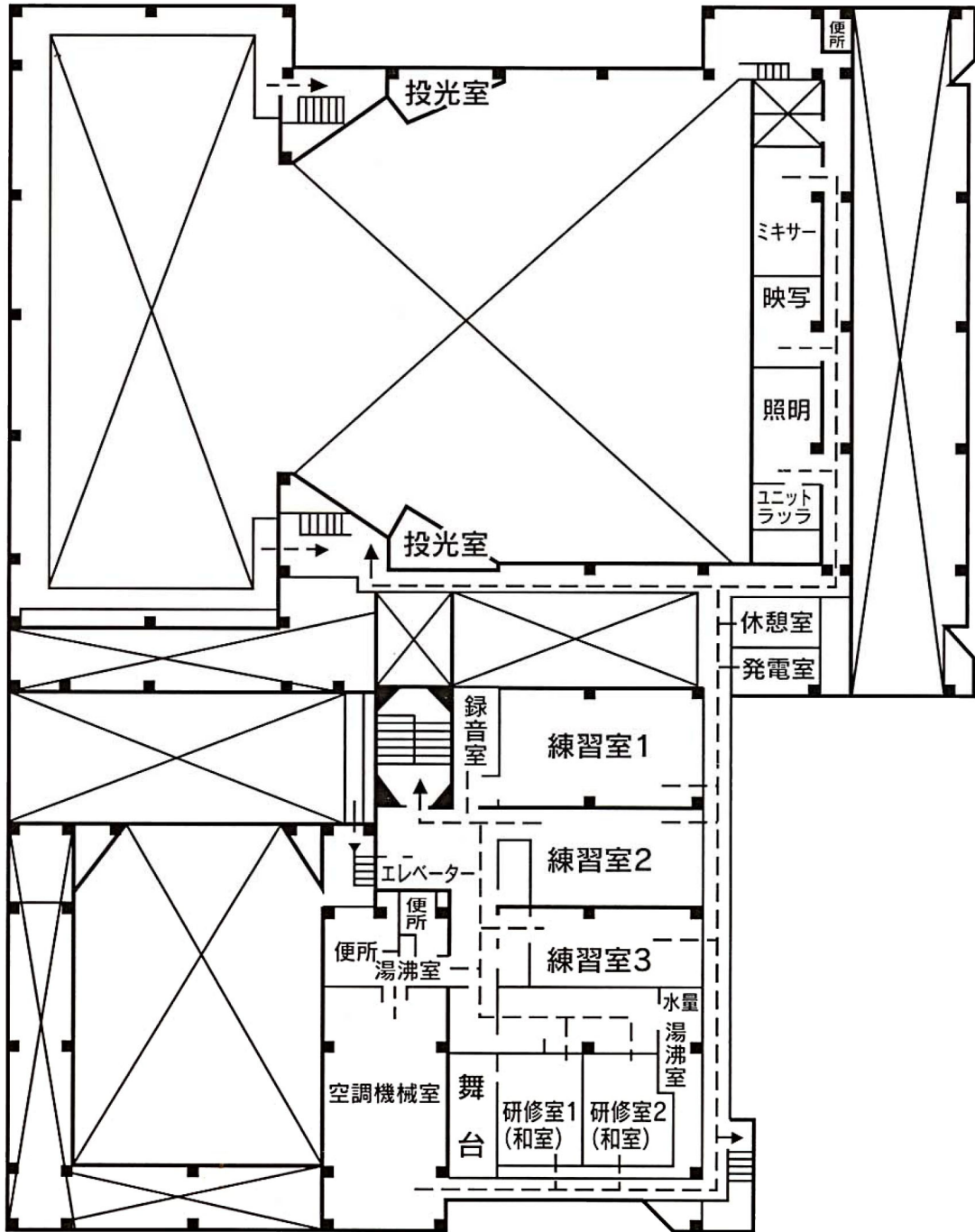
三階平面図 (点線は避難経路)
